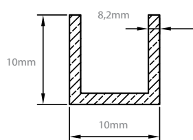
Προφίλ Π για σταθερά ντουζιέρας Εσωτερικό κενό 8,2mm RMB-713
