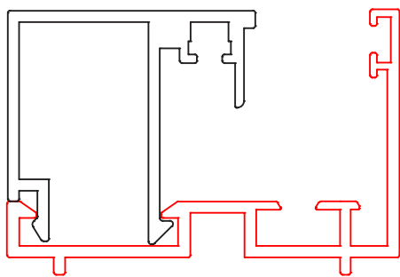
Προφίλ Π για σταθερά ντουζιέρας Εσωτερικό κενό 13mm RMB-712
